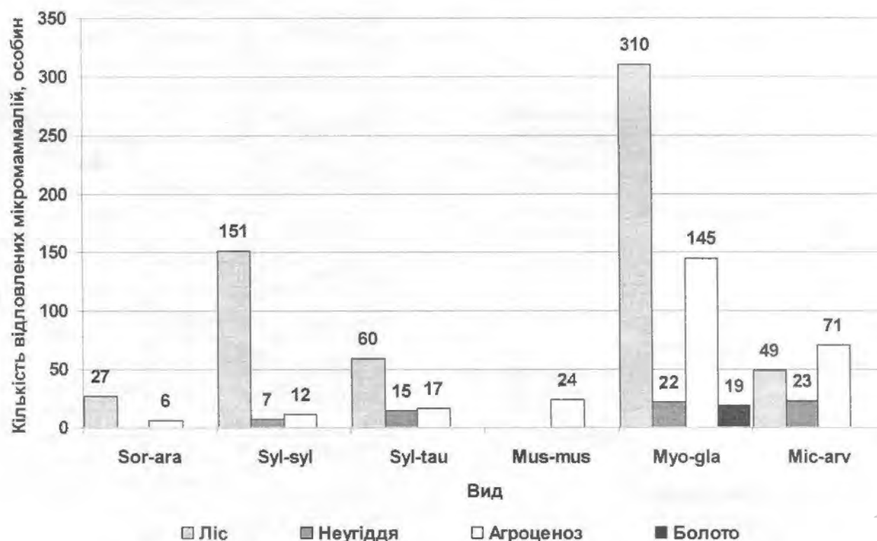
Рис. 2. Біотопічний розподіл кількості виловлених мікромамалій за 2006-2007 роки (в підписах використано акроніми латинських назв видів)
